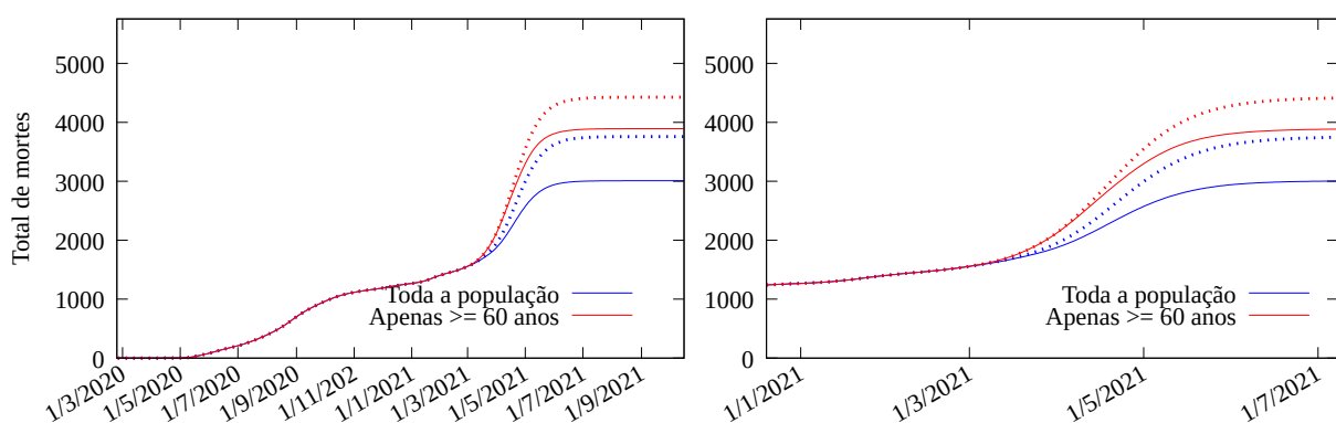
Figura 7: Modelo ajustado até o presente e prognósticos: total de mortes no Tocantins por COVID-19. O gráfico à direita é uma ampliação sobre o ano de 2021. A linha contínua em azul corresponde ao cenário em que toda a população é vacinada, começando pelos mais velhos (95% de eficácia linha contínua e 70% de eficácia linha pontilhada). A linha em vermelho corresponde ao cenário em que apenas pessoas com 60 anos ou mais de idade são vacinadas (95% de eficácia linha contínua e 70% de eficácia linha pontilhada).
