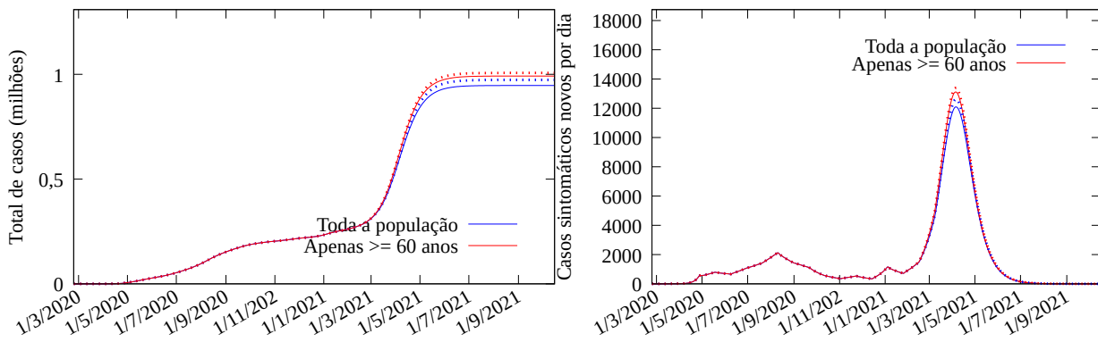
Figura 8: Esquerda: Modelo ajustado até o presente e prognósticos: estimativa do total real de casos sintomáticos no Tocantins . Direita: casos sintomáticos novos por dia.
